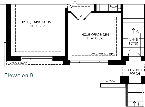
Elevation B
